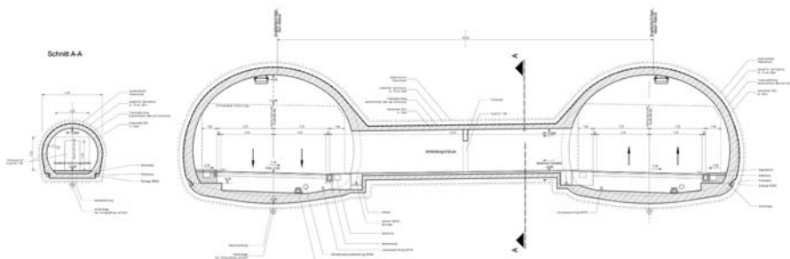
begehbarer Verbindungsstollen
